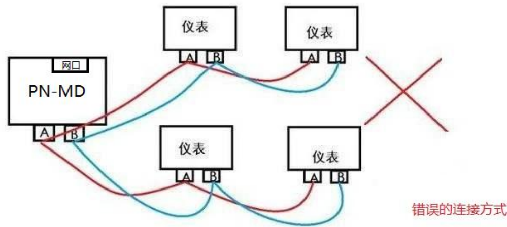
RS485总线组网接线图
